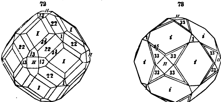
Amalgam.
